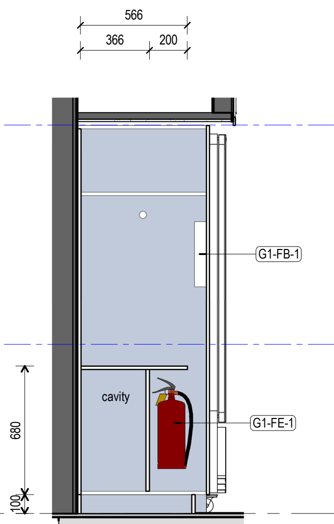
7 Detail 8 1 : 20
