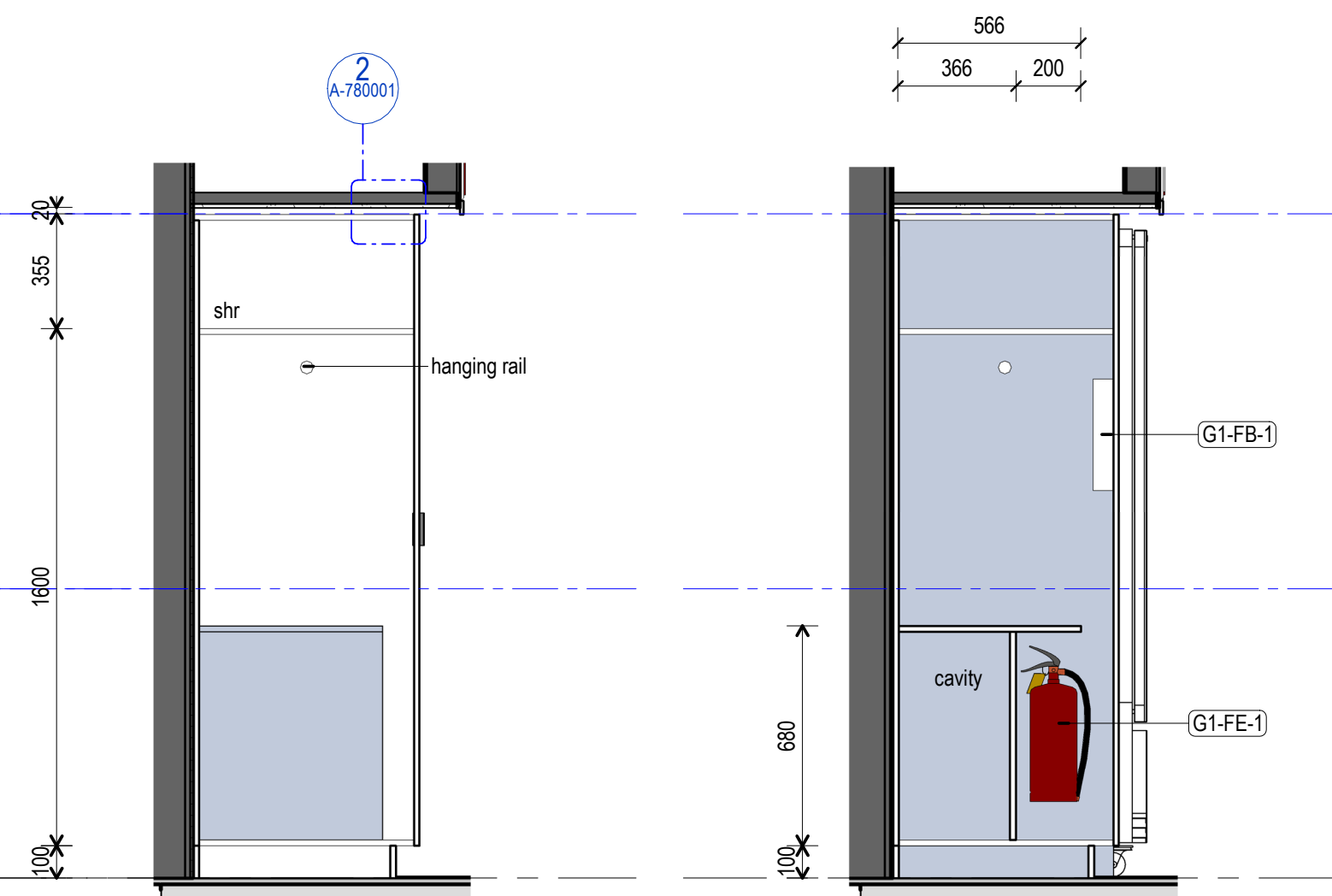
4 JO-ST-2 Section 1 1 : 20
