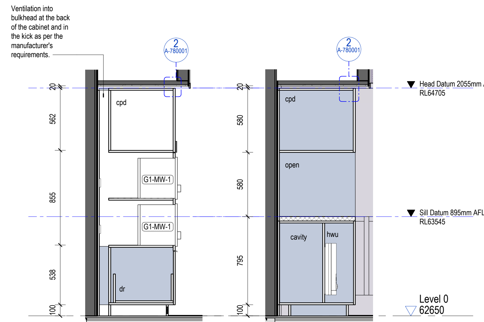
5 JO-ST-2 Section 2 1 : 20
